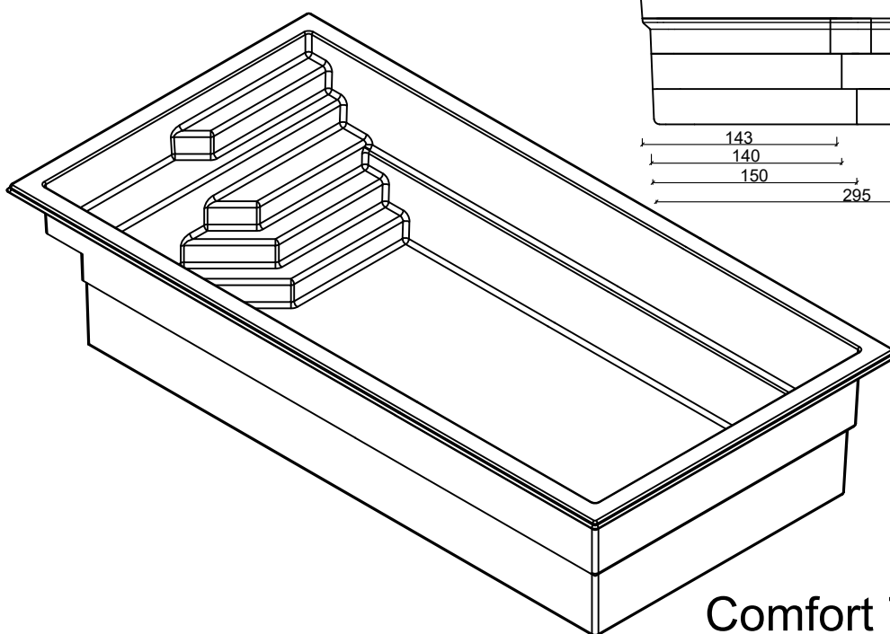
Widok
