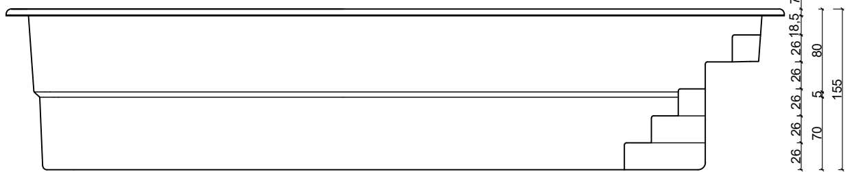
Przekrój B-B'
