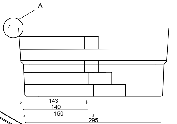
Przekrój B-B'
