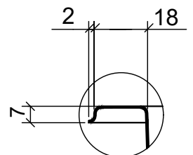
Szczegół A
