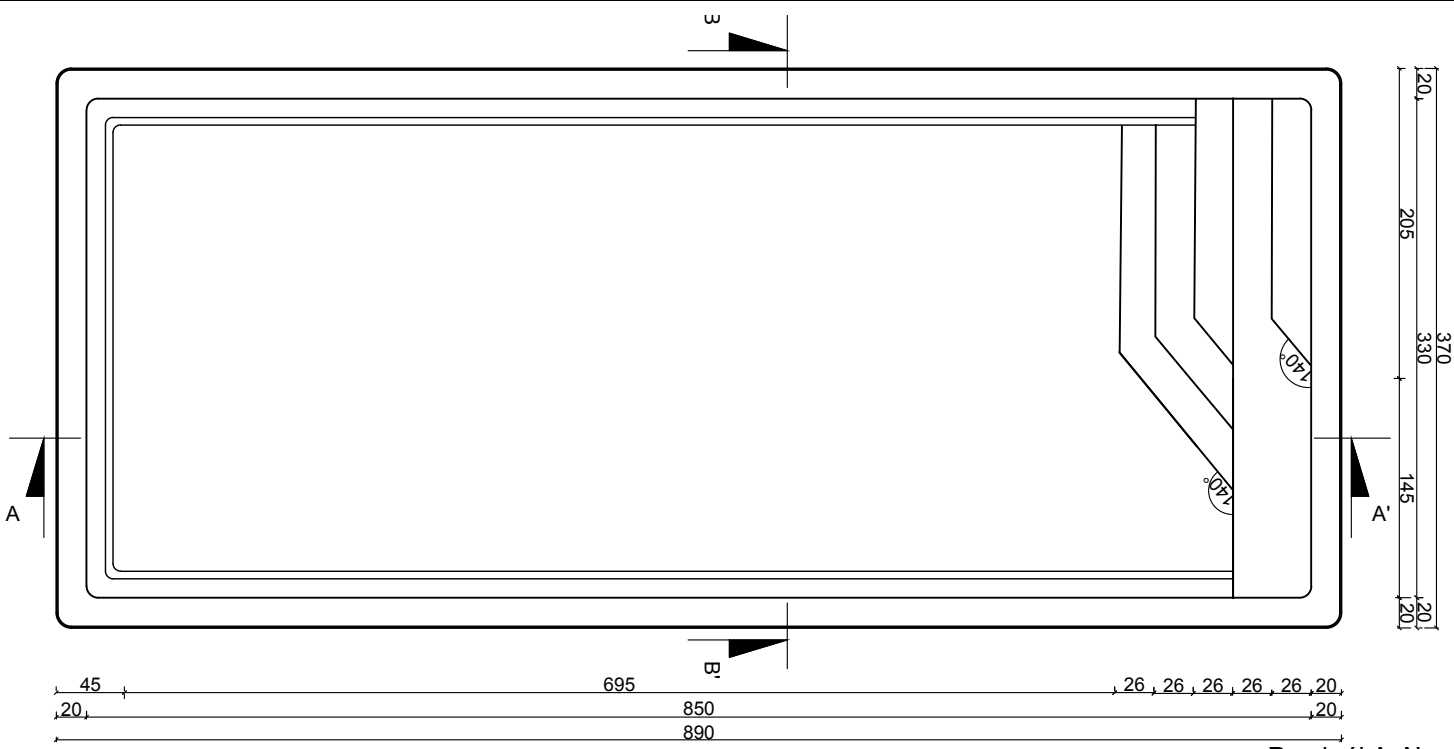
Przekrój A-A'
