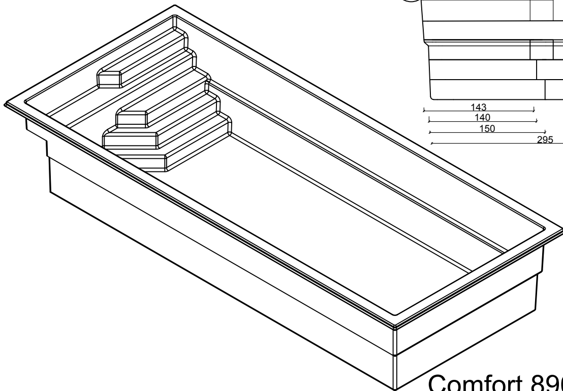
Widok
