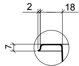
Szczegół A
