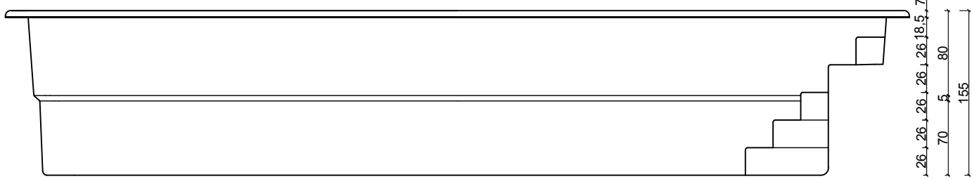
Przekrój B-B'
